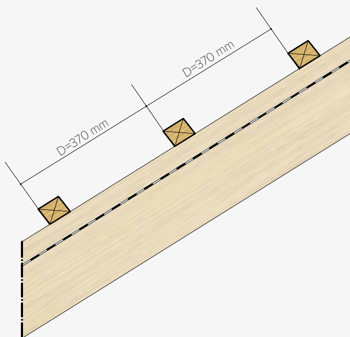
Lektavstand (D) for Decra Elegance-takpanner er 370 mm
